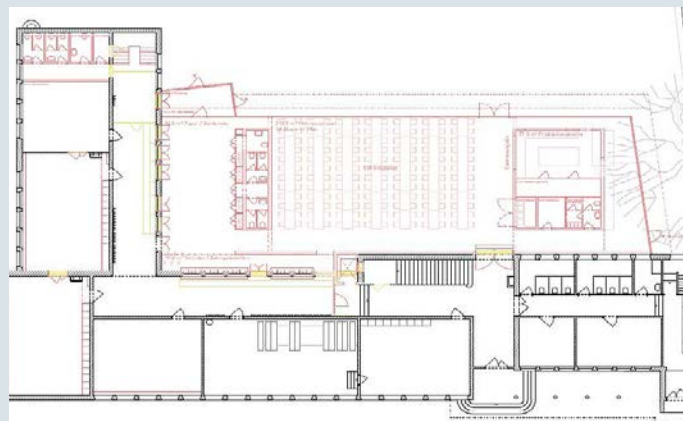
geplante Erweiterung / Anpassung Schulhaus Letten (provisorischer Plan)
